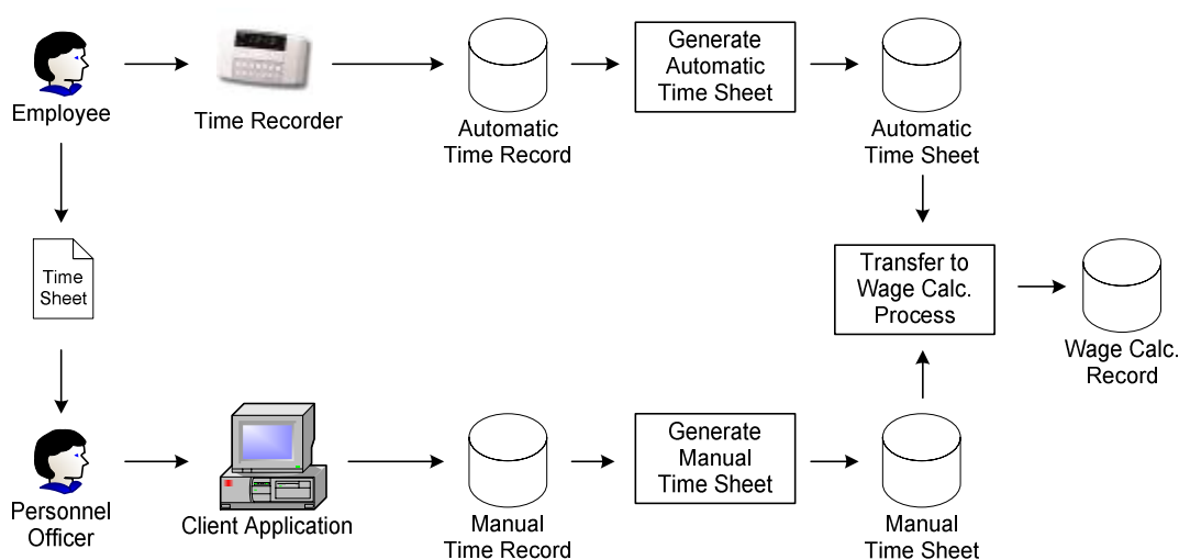
รูปที่ 1.12 โครงสร้างของข้อมูลเวลาทำงาน
