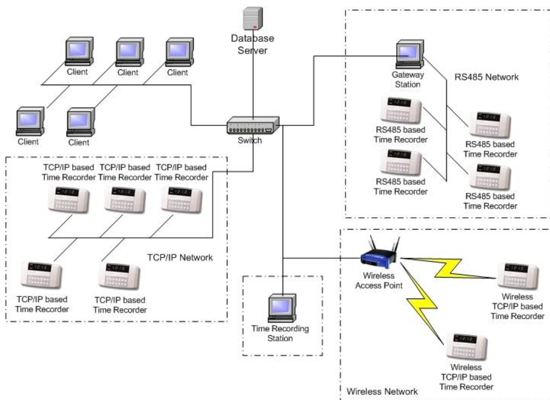
รูปที่ 1.2 เครือข่ายของระบบบันทึกเวลาและบริหารงานบุคคล
