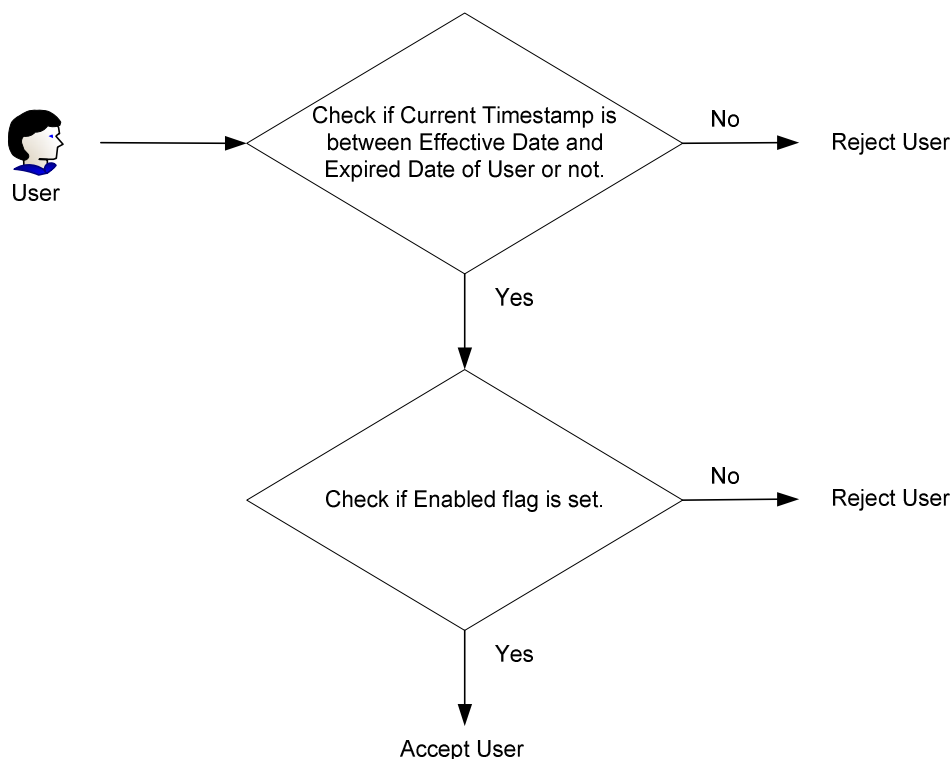
รูปที่ 1.8 กระบวนการตรวจสอบผู้ใช้ของระบบรักษาความปลอดภัยภายใน
