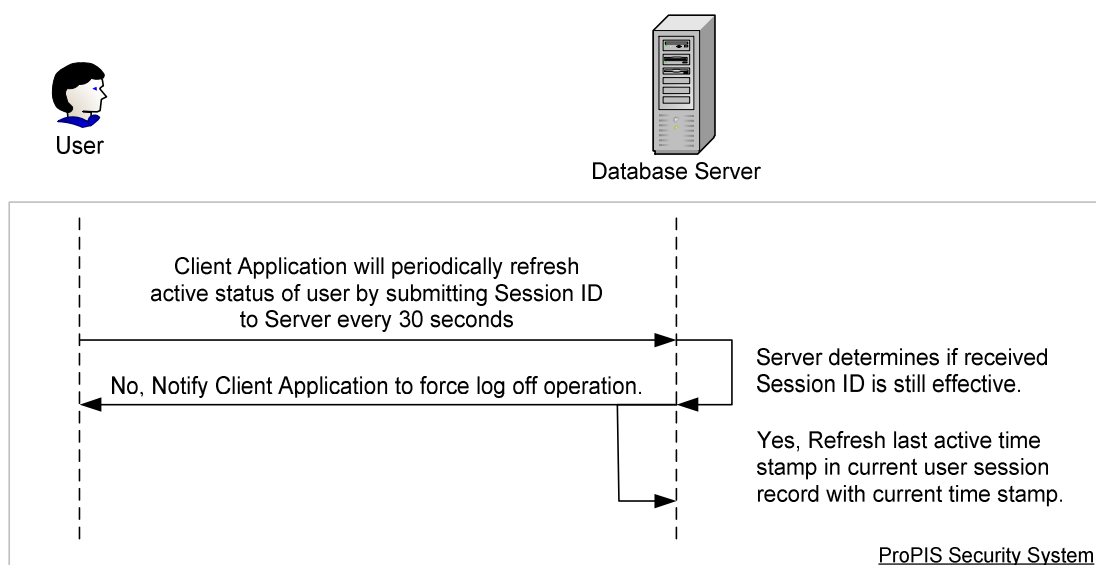
รูปที่ 1.5 กระบวนการยืนยันการเชื่อมต่อระหว่างผู้ใช้กับฐานข้อมูล
