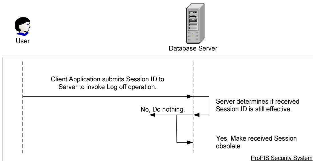
รูปที่ 1.7 กระบวนการยุติการเชื่อมต่อระหว่างผู้ใช้กับฐานข้อมูล
