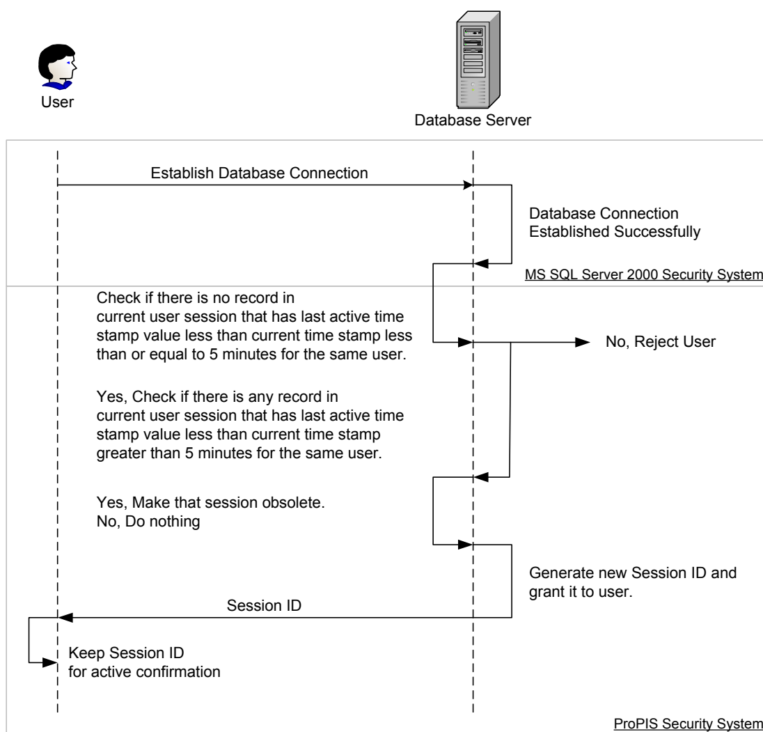
รูปที่ 1.6 กระบวนการเริ่มต้นการเชื่อมต่อระหว่างผู้ใช้กับฐานข้อมูล กรณีไม่ได้ยุติการเชื่อมต่ออย่างถูกต้องในการเชื่อมต่อครั้งก่อน
